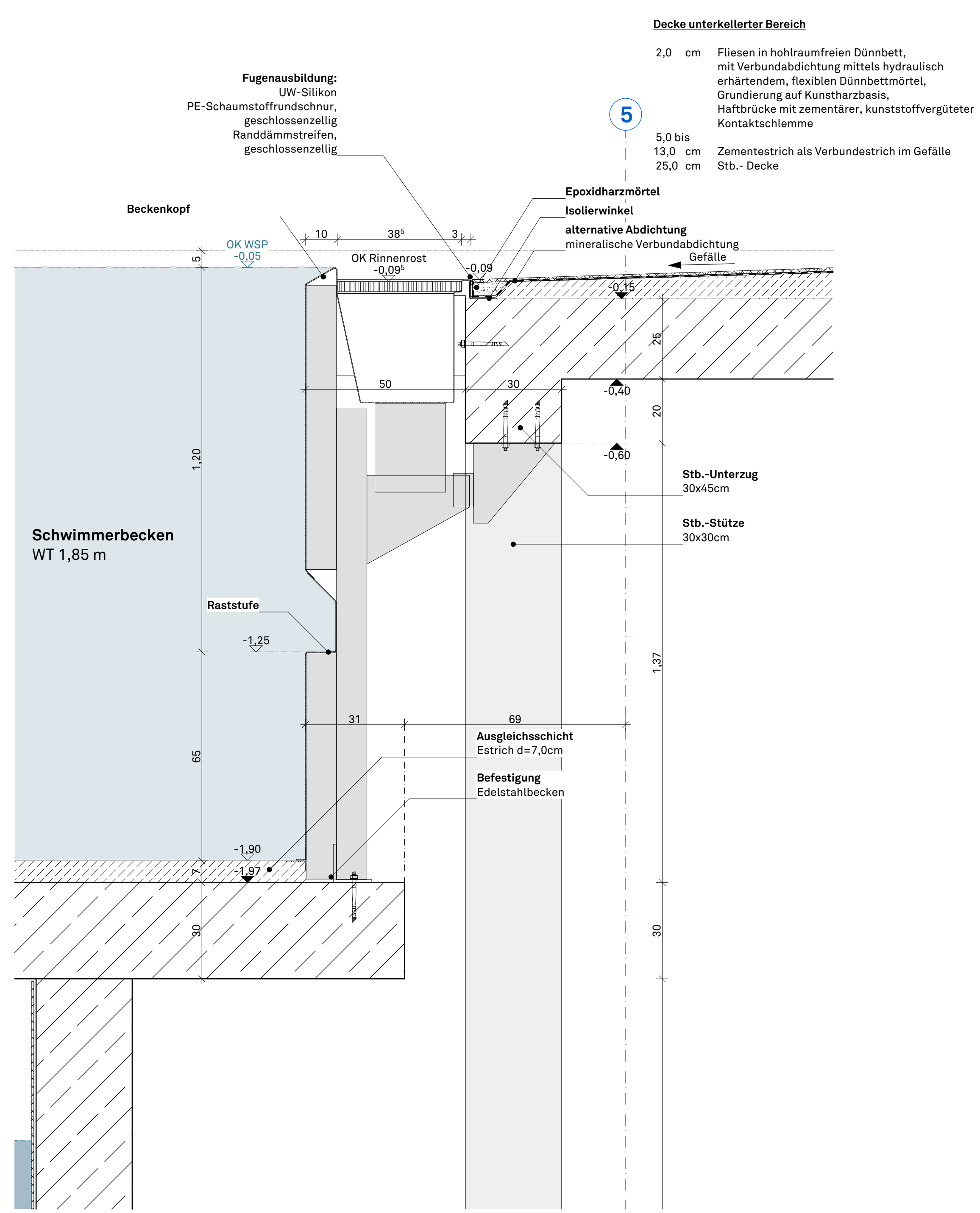
DETAIL 1:10 Schwimmerbecken WT 1,80m
