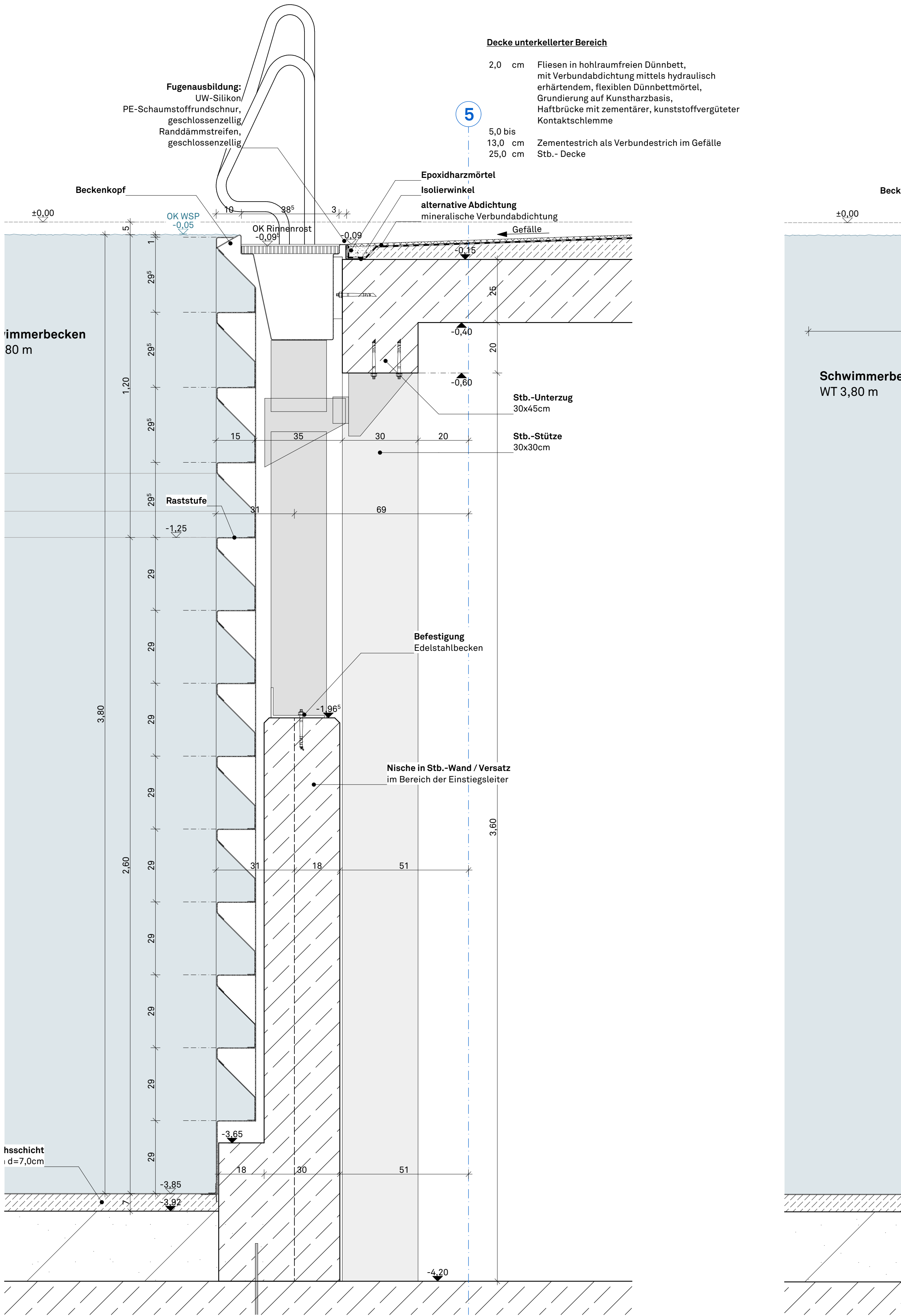
DETAIL 1:10 SB Beckenleiter / Wand WT 3,80m
