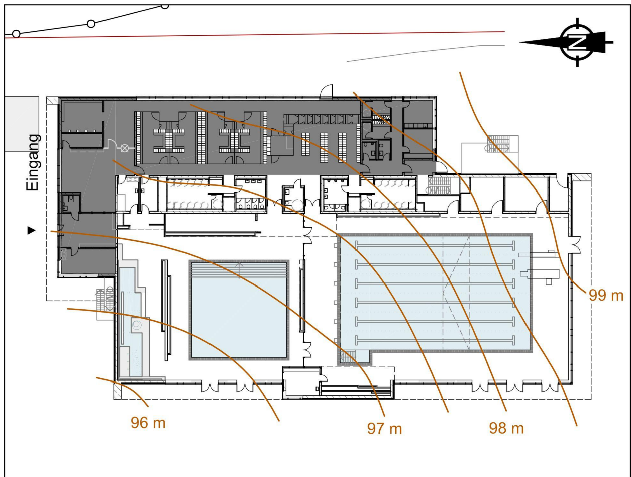
Abb. 1: Schematische Darstellung der Streichlinien der Oberkante der Verwitterungszone
