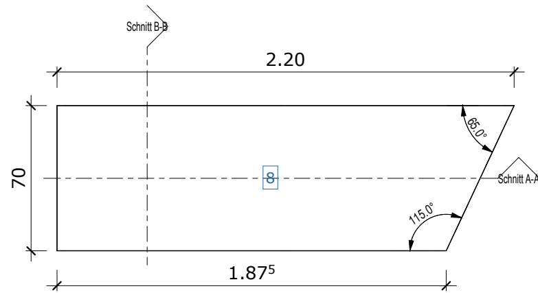
Grundriss
