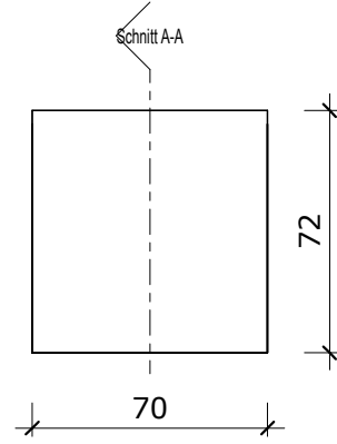
Seiten-Ansicht
