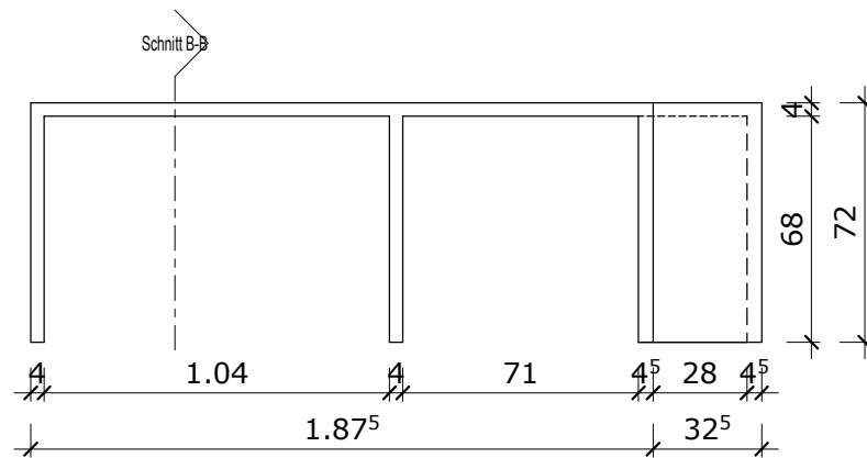
Schnitt A-A
