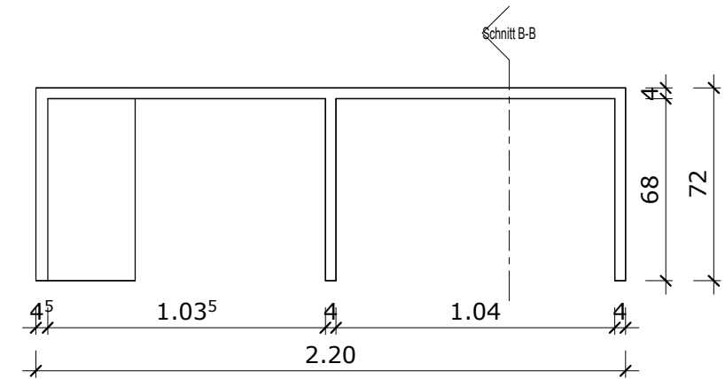
Rück-Ansicht
