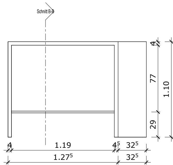
Vorder-Ansicht
