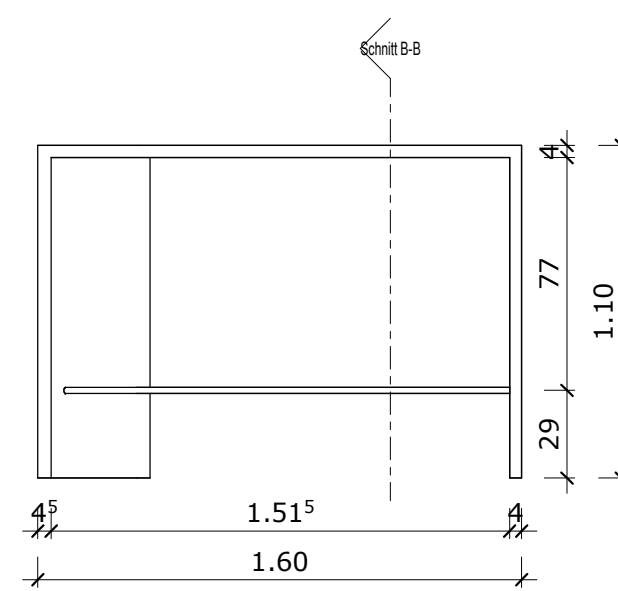
Rück-Ansicht
