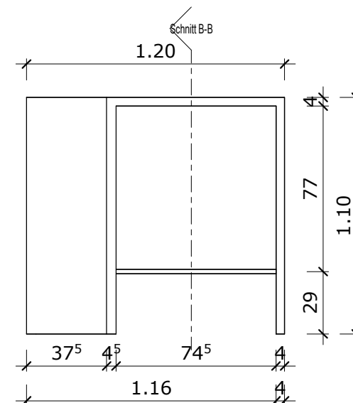
Rück-Ansicht
