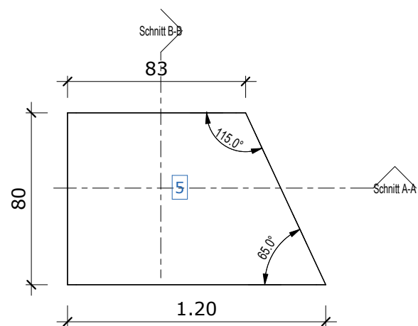
Grundriss
