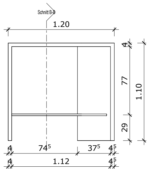
Vorder-Ansicht
