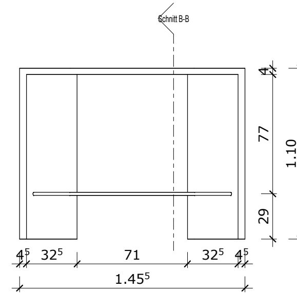
Rück-Ansicht
