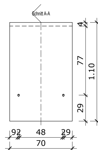
Schnitt B-B
