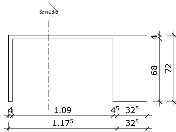
Vorder-Ansicht
