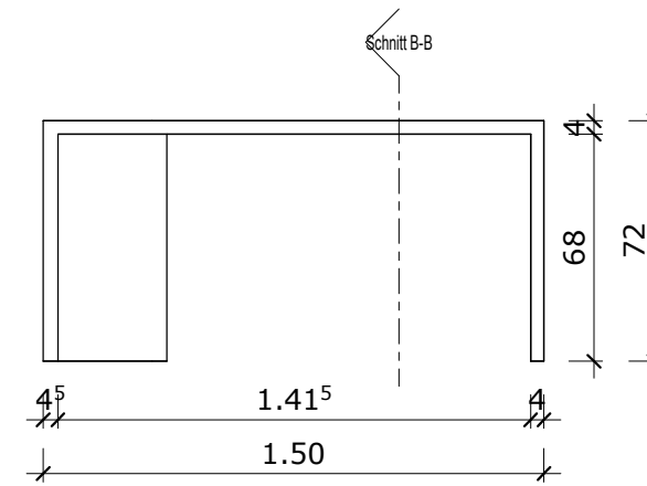
Rück-Ansicht
