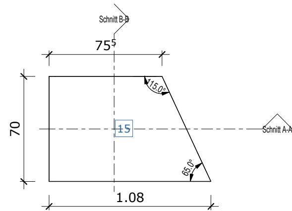
Grundriss
