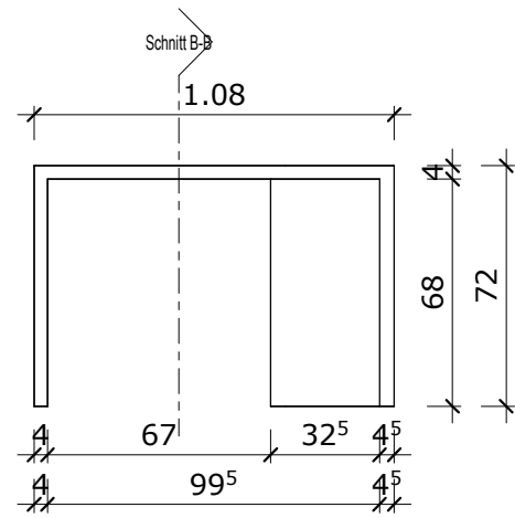
Vorder-Ansicht
