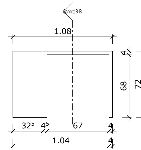
Rück-Ansicht
