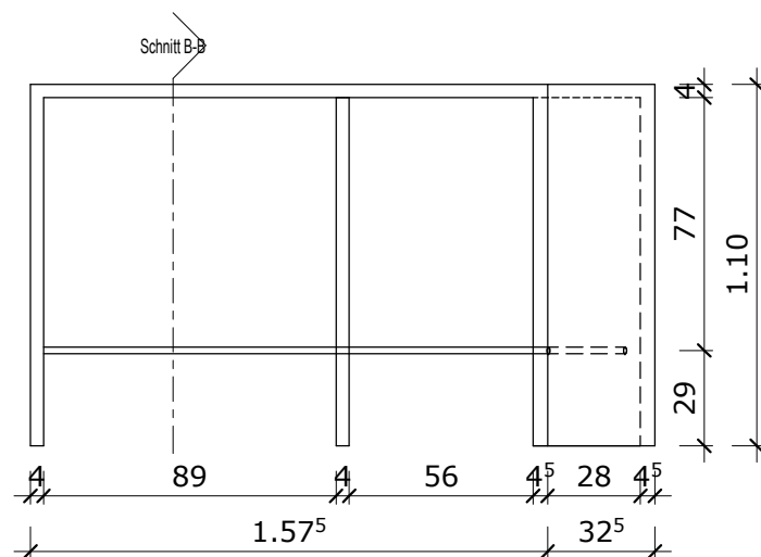
Schnitt A-A
