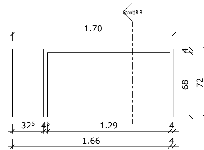
Rück-Ansicht
