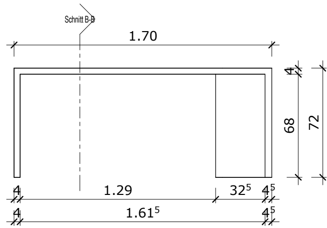
Vorder-Ansicht
