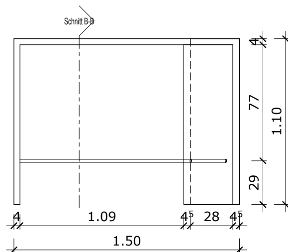
Schnitt A-A
