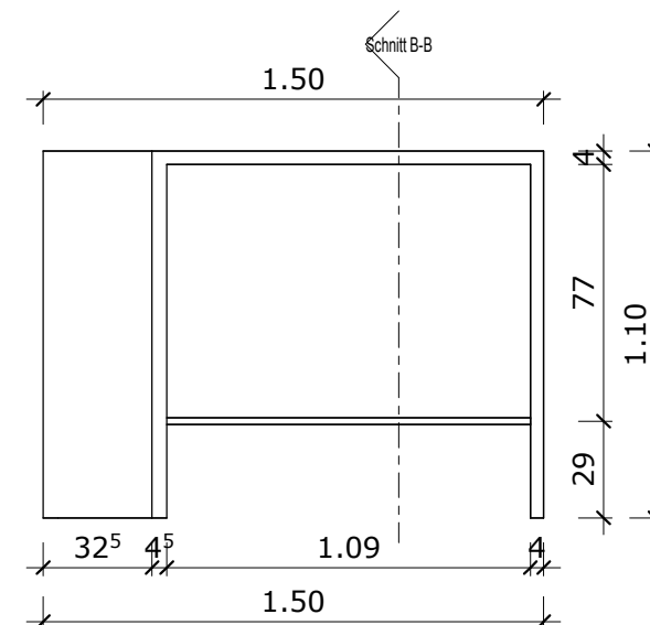
Rück-Ansicht
