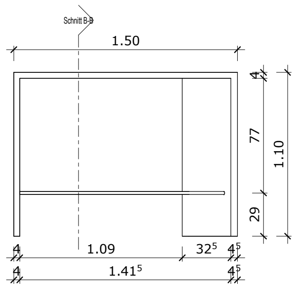
Vorder-Ansicht
