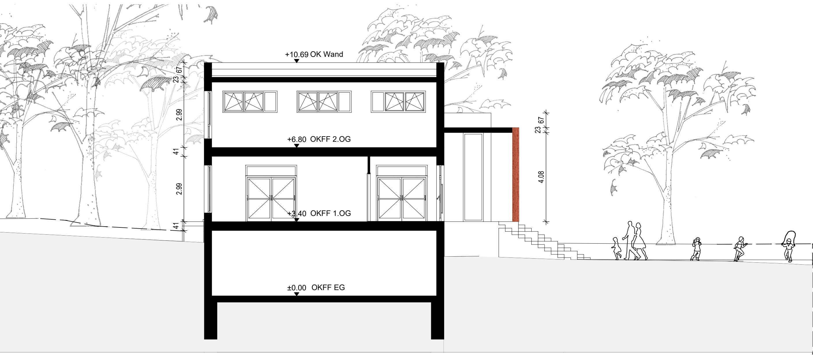
SCHNITT D-D M. 1:100
