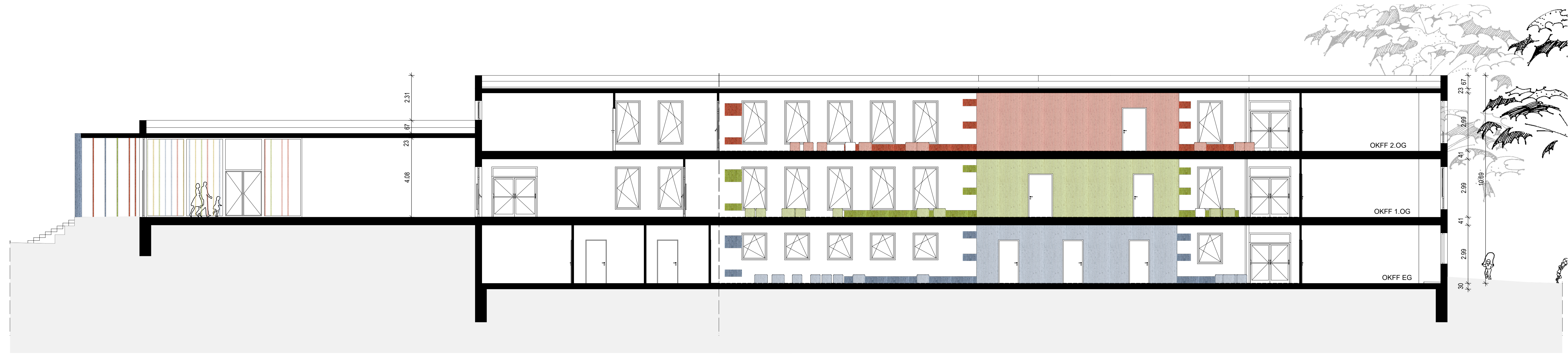
SCHNITT A1-A1 + A2-A2 M. 1:100
