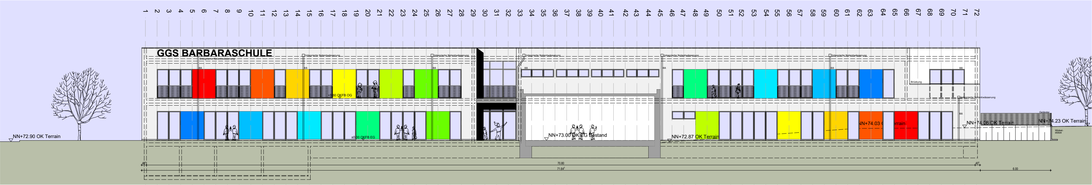
Ansicht Süd-West
