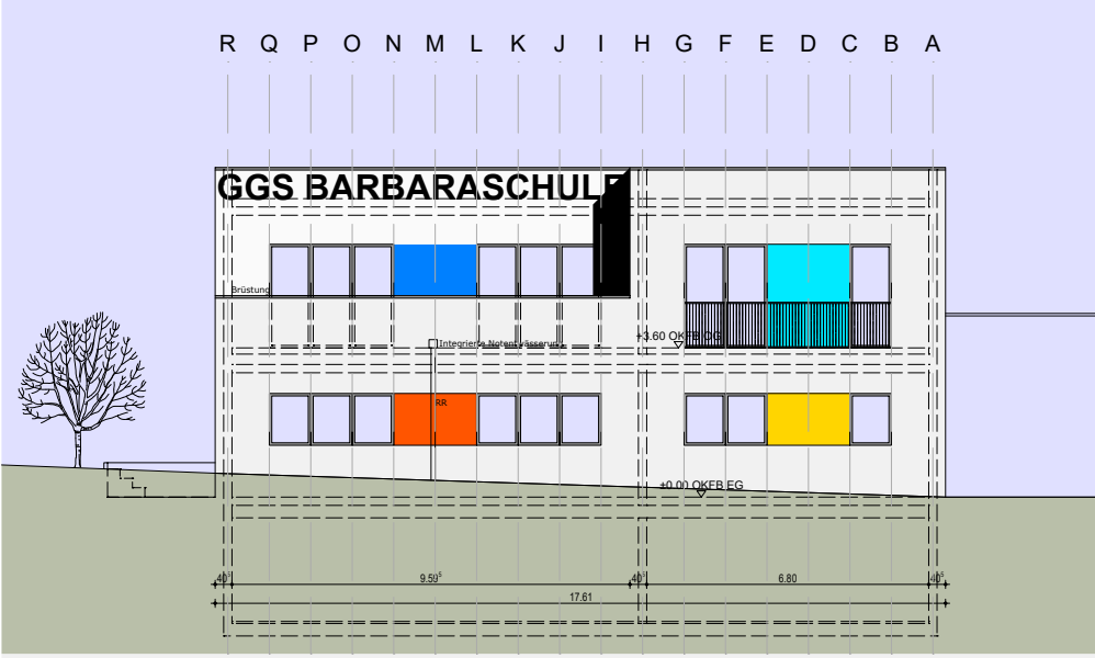
Ansicht Nord-West
