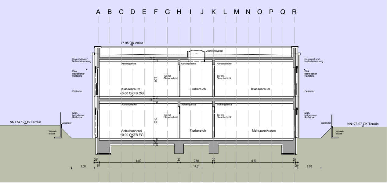
Querschnitt B-B
