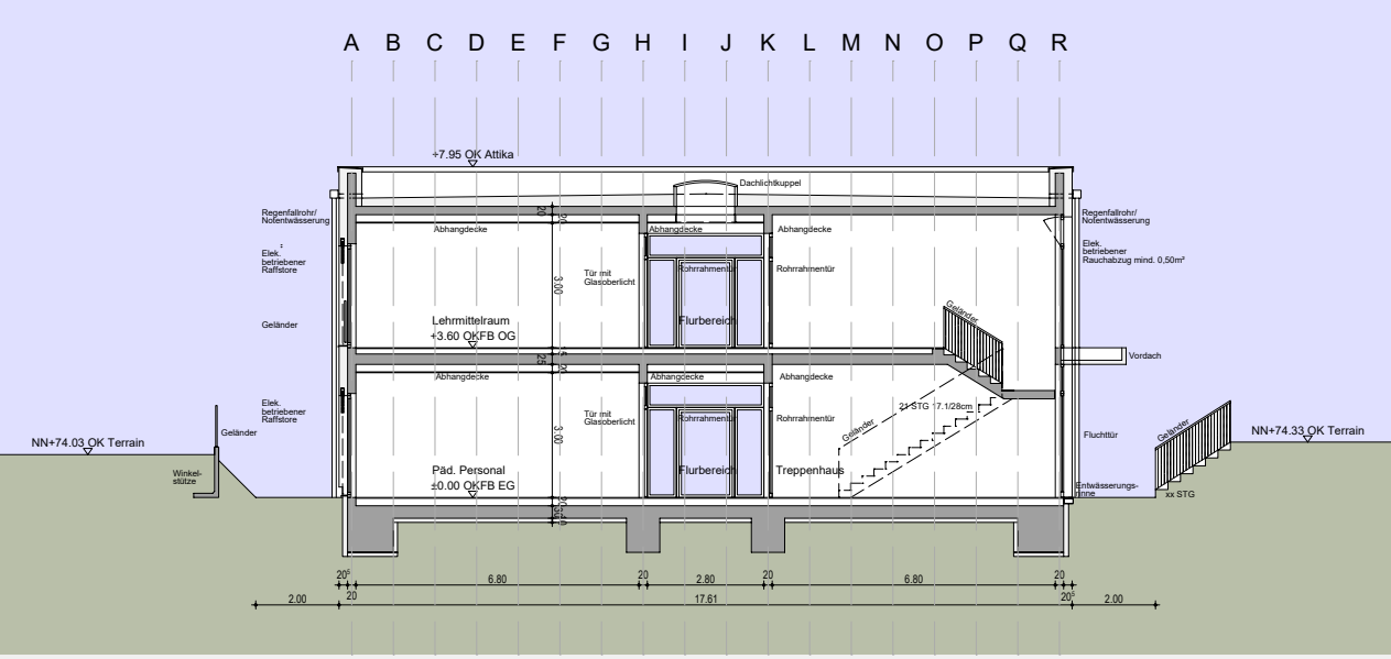
Querschnitt A-A
