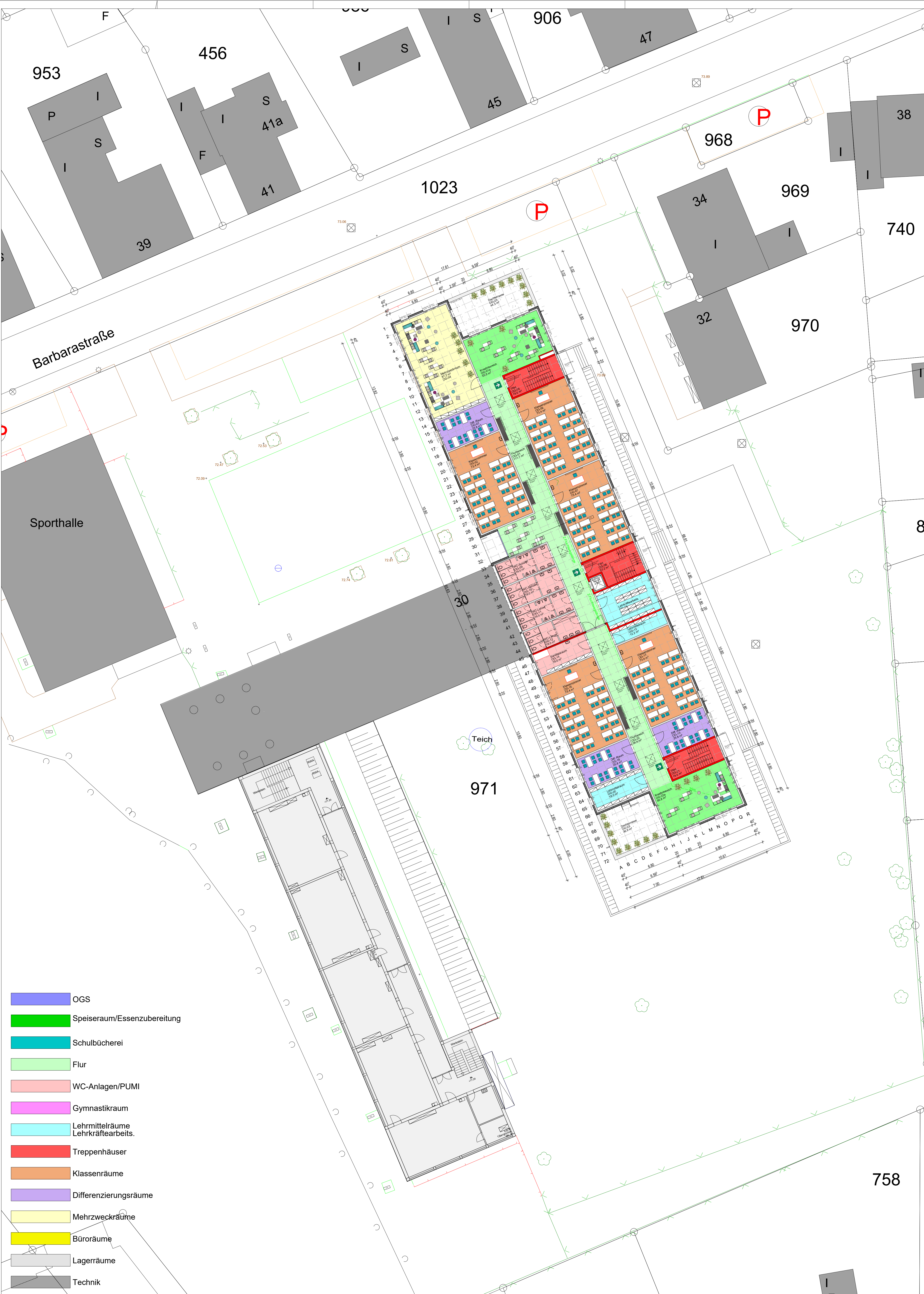
GGs Barbaraschule- Variante C.2 Grundriss Obergeschoss M 1-200 Stand 05.06.2023 Jäger Gerull Architekten PartGmBb 40215 Düsseldorf Kirchfeldstrasse 82A
