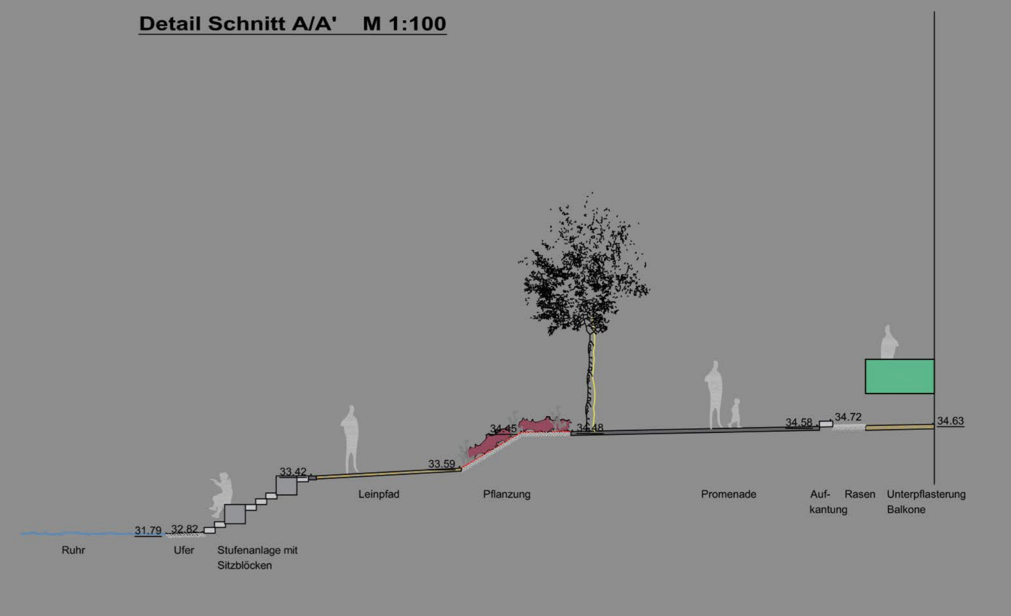
Detail Schnitt A/A' M 1:100
